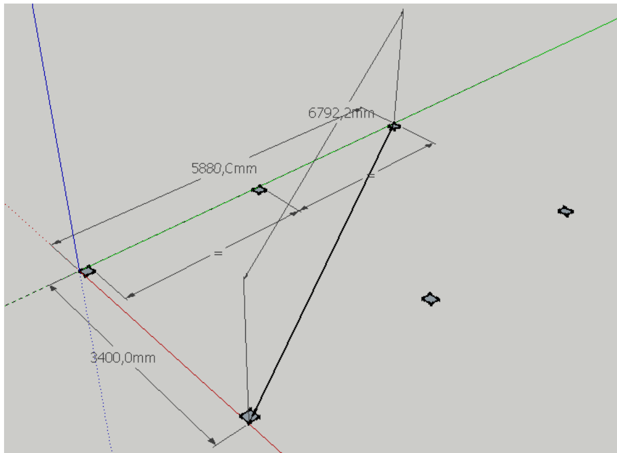
Figure 1 - Cotes d'Implantation
