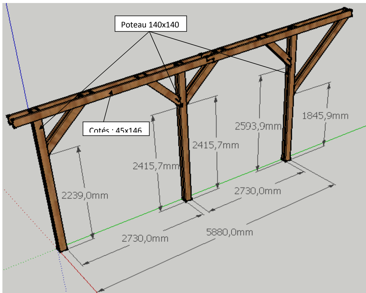
Figure 2: Coté assemblé avec principales cotes
